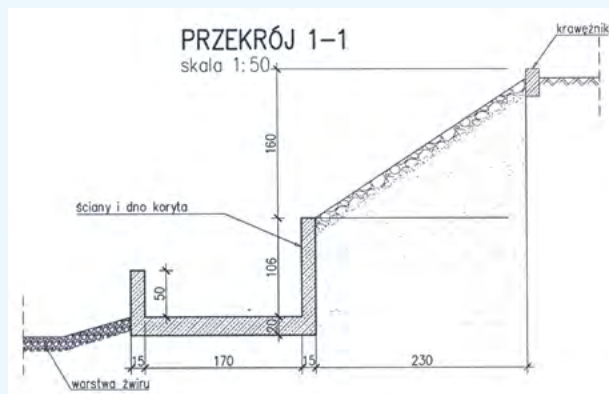
Przekrój poprzeczny koryta skarpy
